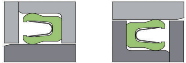
(Fig:4-1) Open groove
